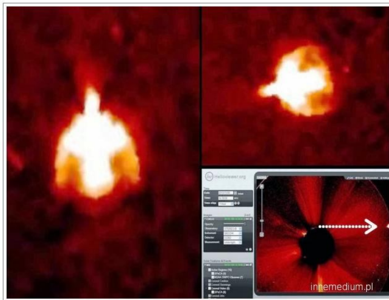
Anielskie UFO w okolicy Słońca
